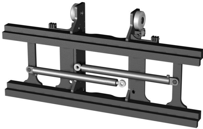
Vogn sideforskyvning/spredning 75-90 B=2000 mm
